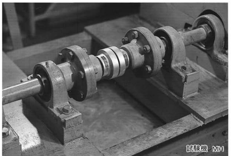
揚水ポンプ MT
